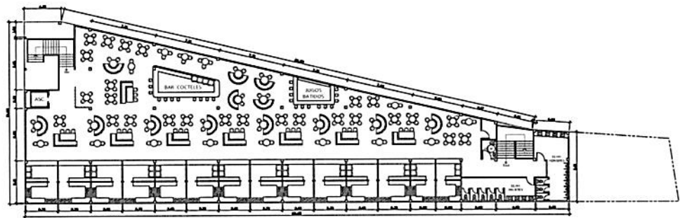
PLANTA ALTA ARQUITECTÓNICA ÁREA DE CONSTRUCCIÓN = 968.00 m 2 Esc. 1:125
